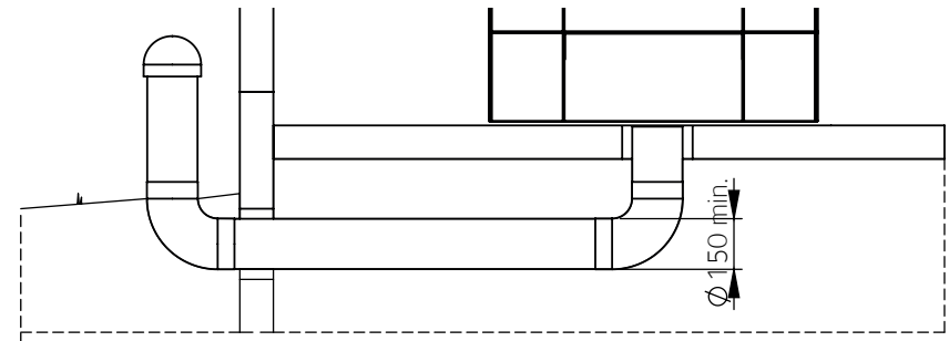
Maanvarainen alapohja
