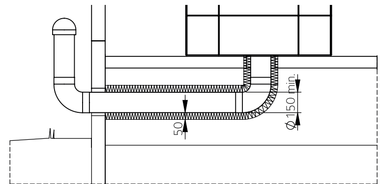
Tuulettuva alapohja
